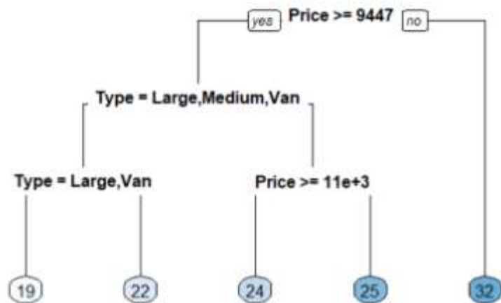
Árbol de regresión
